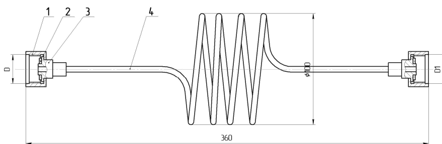
Рис.1 Змеевик ЗМК ДЖЕТ 133 00 00 00, -01, -02, -04, -11, -12, -13
