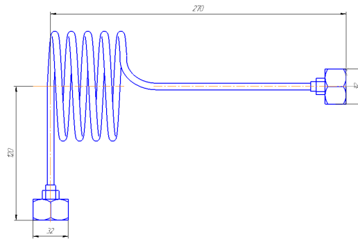
Рис.3 Змеевик ЗМК ДЖЕТ 133 00 00 00-33, -43
