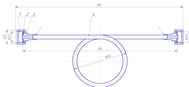
Рис.1 Змеевик ЗМК ДЖЕТ 133 00 00 00, -01, -02, -04, -11, -12, -13
